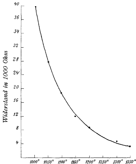
Fig. 16. Baryt.
