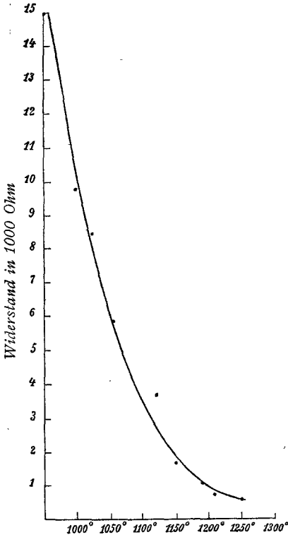
Fig. 8. Rauchquarz B.
