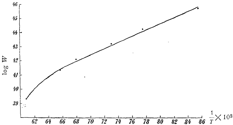
Fig. 12. Chrysoberyll.
