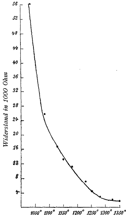
Fig. 14. Topas.
