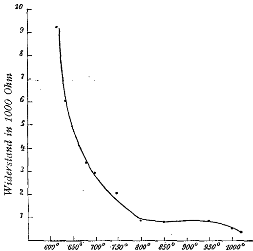
Fig. 13. Granat.
