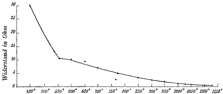
Fig. 18. Wolframit.
