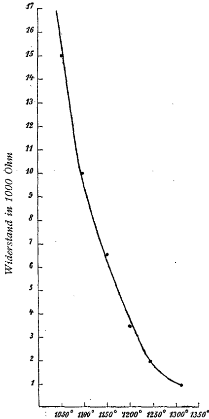
Fig. 7. Rauchquarz A.
