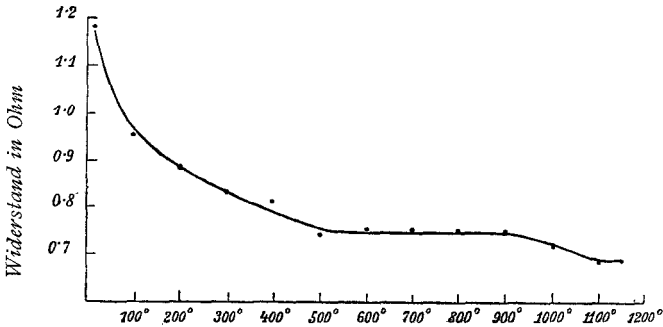
Fig. 11. Magneteisen.
