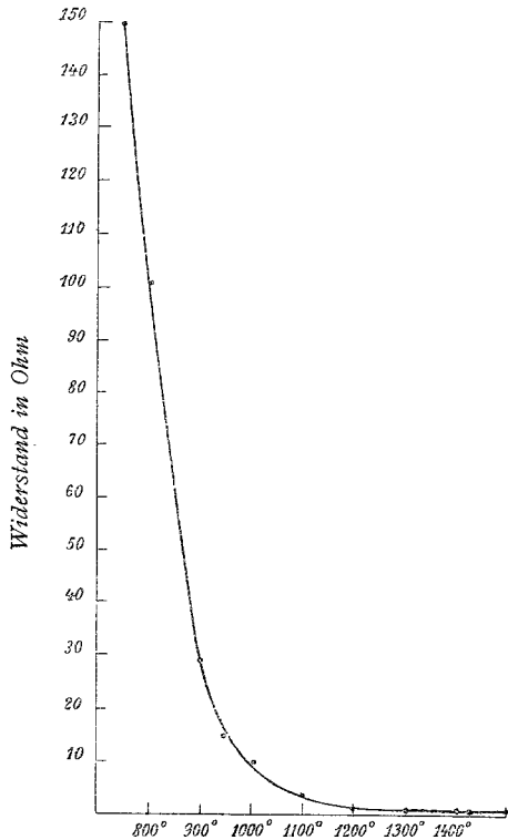
Fig. 1. Zinnstein.
