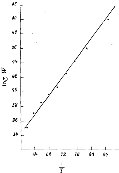
Fig. 17. Baryt.
