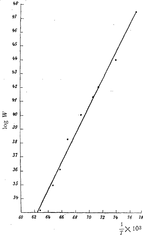
Fig. 15. Topas.
