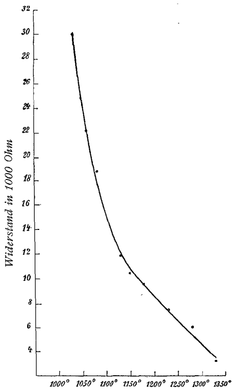
Fig. 9. Saphir.
